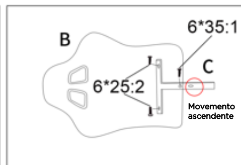
3. Instale a barra em T no chassi do encosto
