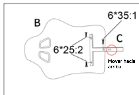
3. Instale la barra en T en el chasis del respaldo
