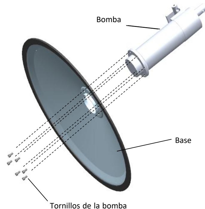
Tornillos de bomba X6
