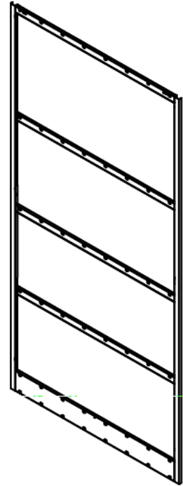
Panel trasero (1 pieza)
