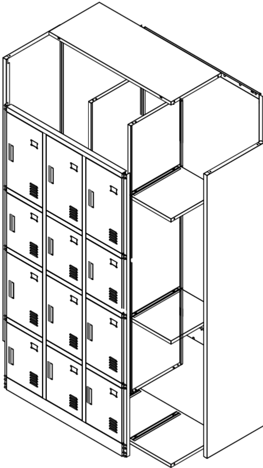
Diagrama esquemático de instalación de doce puertas
