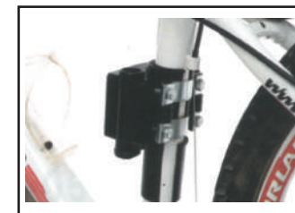
9. Instale na linha de freio
